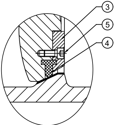
FIG. 3 Detail Y
